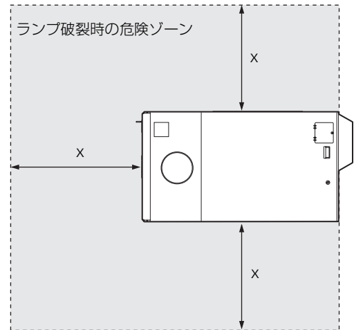
上面図
